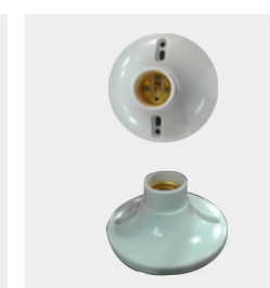
Cod.: VC090071 PORTALAMPARA PORCELANA E27 C/ PUENTE 5/8 Cod.: VC002710 PORTALAMPARA E27 PLAFONIER PLASTICO BLANCO
