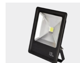
PROYECTOR LED 10W 4000K 88-264V IP65
