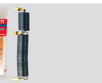
Cod.: L0589104 RESISTENCIA DUCHA DUO SHOWER 220V 6800W
